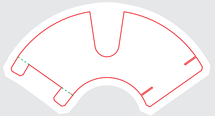
Schablone für den Abdampf-Konus aus Aluminiumblech
